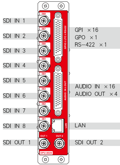
DPU-8020 背板接口说明
