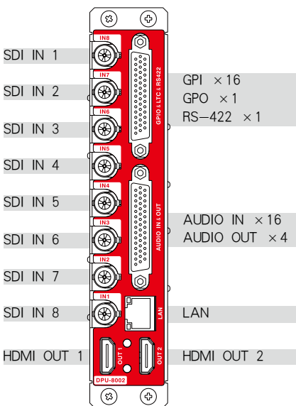
DPU-8002 背板接口说明
