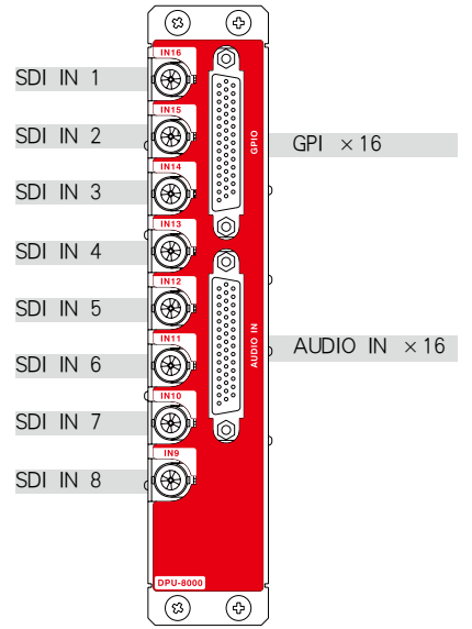
DPU-8000 背板接口说明
